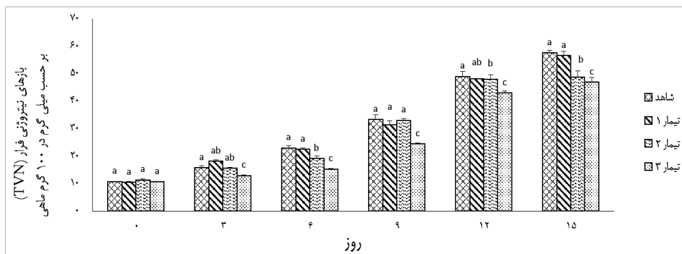
نمودار (۴) - میزان تغییرات TVB-N در تیمارهای مختلف پوشش خوراکی نشاسته ذرت و اسانس فلفل سیاه در بسته‌بندی تحت خلأ در فیله کپور نقره‌ای در دمای یخچال. حروف کوچک غیر هم‌نام نشان دهنده اختلاف معنی‌دار در سطح (P < 0.05) می‌باشد.
