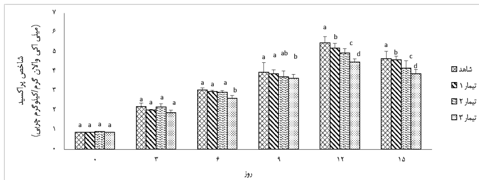
نمودار ۲- میزان تغییرات PV در تیمارهای مختلف پوشش خوراکی نشاسته ذرت و اسانس فلفل سیاه در بسته‌بندی تحت خلأ در فیله کپور نقره‌ای در دمای یخچال. حروف کوچک غیر هم‌نام نشان‌دهنده اختلاف معنی‌دار در سطح P < 0/05 می‌باشد.
